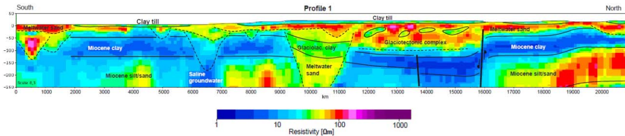
Figur 6.1 Eksempel på SkyTEM-kortlægning ved Tønder. Fra Jørgensen et al. 2015.
