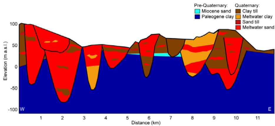
Figur 7.6: Konceptuel profilskitse for modelområdet ved Kasted (fra Høyer et al. 2015).
