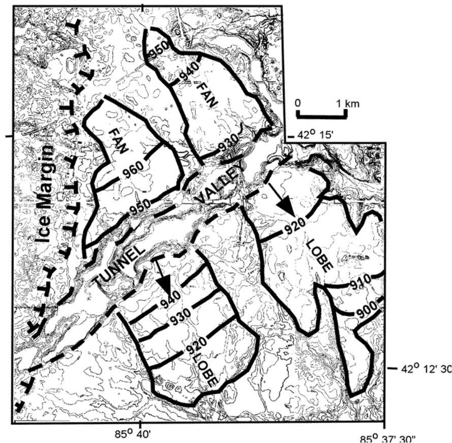
Figur 8.6: Eksempel på en åben tunneldal fra Michigan, USA. Dalen har været udfyldt med dødis under dannelsen af to smeltevandssletter. Ved afsmeltingen af dødisen er smeltevandsslettens aflejringer kollapsede og dalen kommet til syne. Modificeret fra Kehew et al. 1999.
