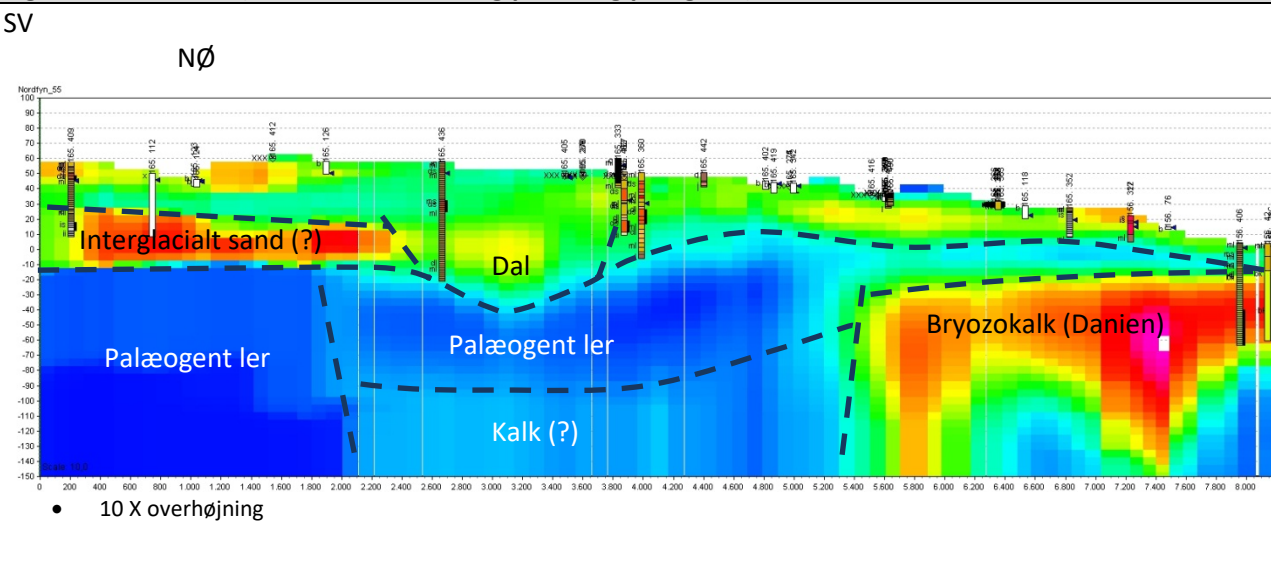
Figur 4: Profilsnit 1 (SV-NØ; se omtrentlig placering på figur 1)
