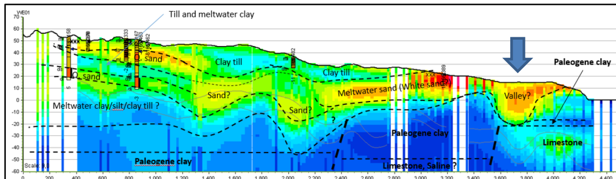
Figur 5: Vertikalt profilsnit 2 (SV-NØ; se omtrentlig placering på figur 1)
